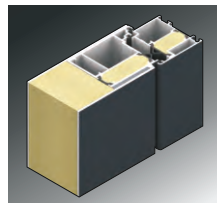
AT 70 flächenbündig
